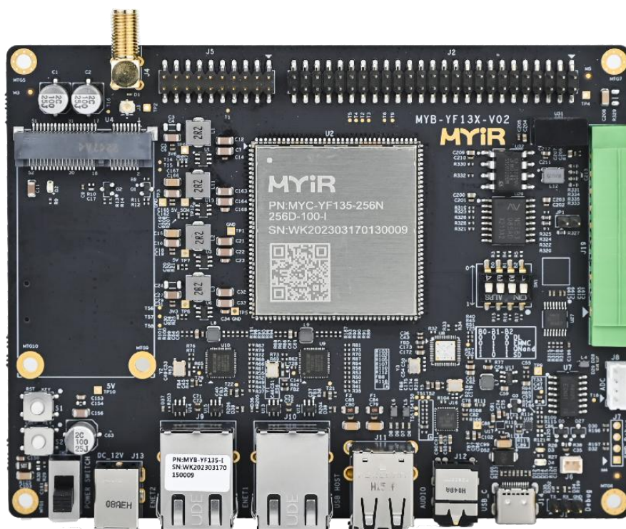
图 1-1 MYD-YF13X 开发板
