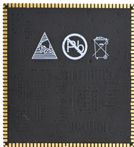
图 3-2 核心板 MYC-YF13X 背面图
