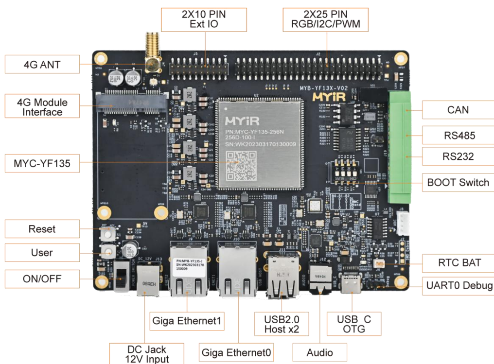
图 4-1 MYD-YF13X 开发板接口正面图
