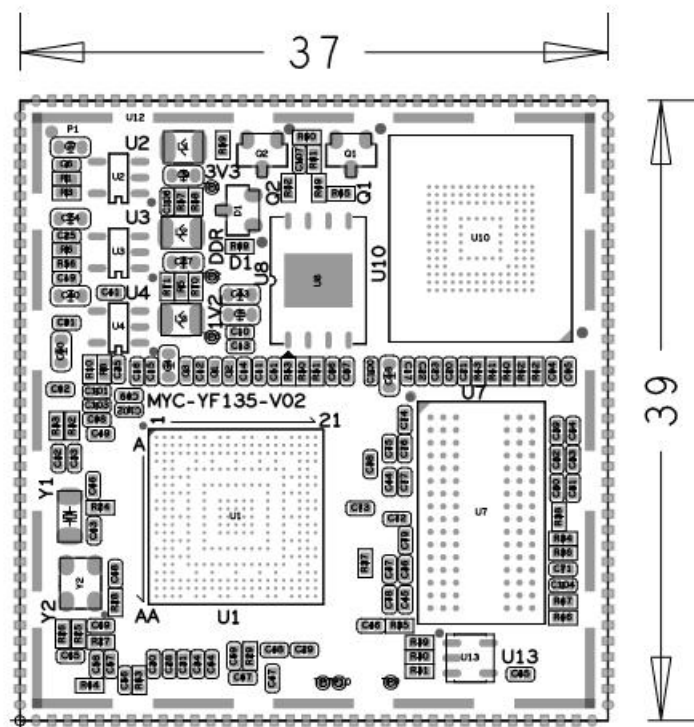
图 3-4 MYC-YF13X 核心板机械结构图 (单位: mm)
