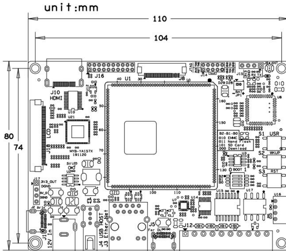
图 9 MYB-YA157C 机械尺寸图
