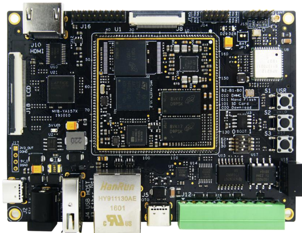
图 1 MYD-YA157C 开发板
