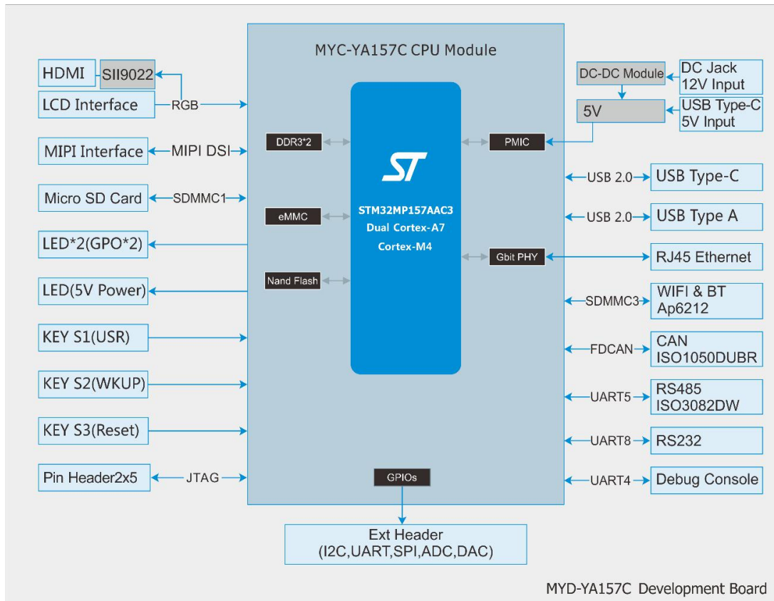
图 8 MYD-YA157C 开发板系统框架图
