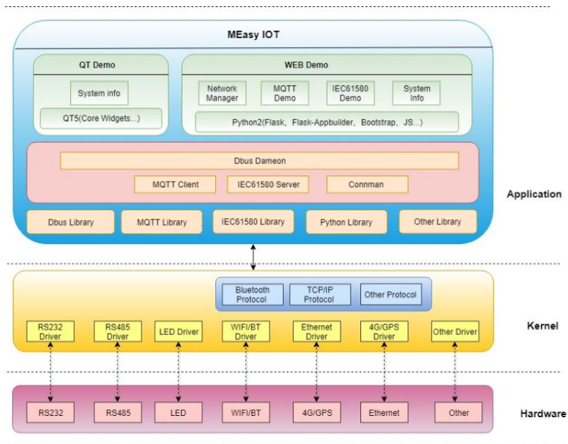
图 11 MEasy IOT 系统框图
