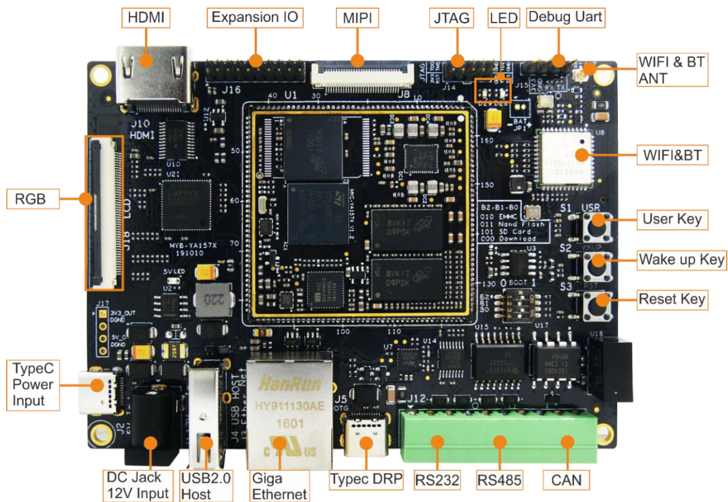
图 7 MYD-YA157C 开发板接口图
