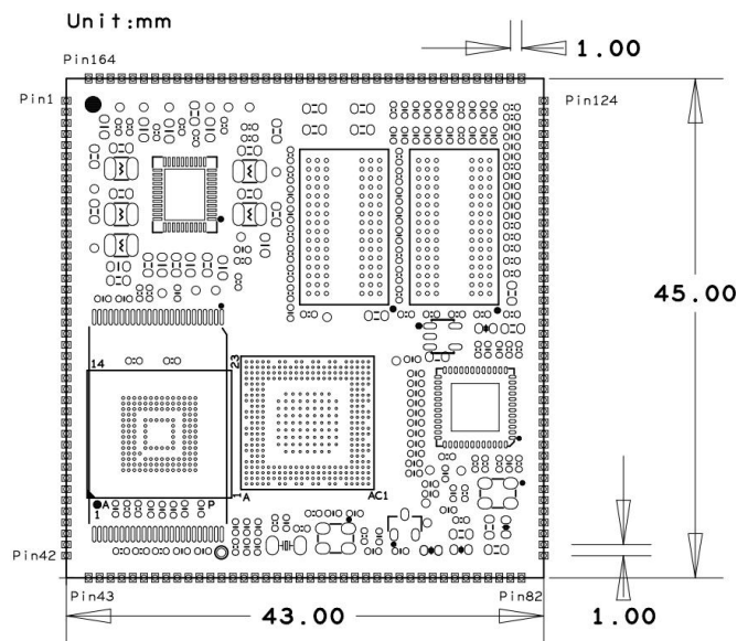
图 6 MYC-YA157C 机械结构图（单位：mm）
