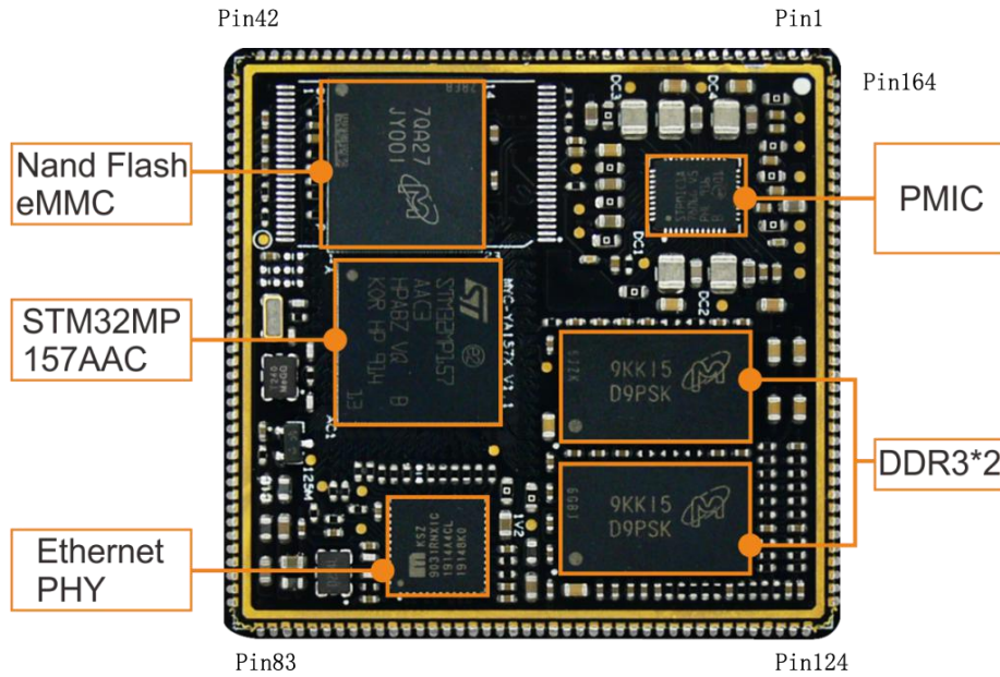
图 4 MYC-YA157C 核心板接口图
