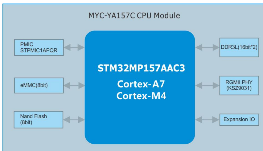
图 5 MYC-YA157C 核心板结构框图
