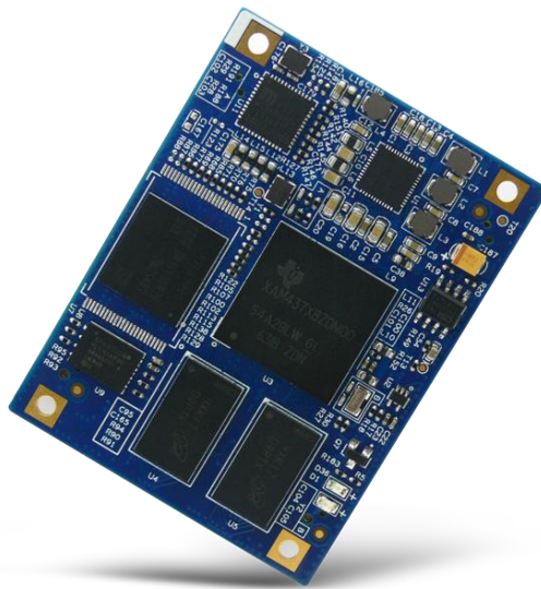
图 1-1 产品正面图
