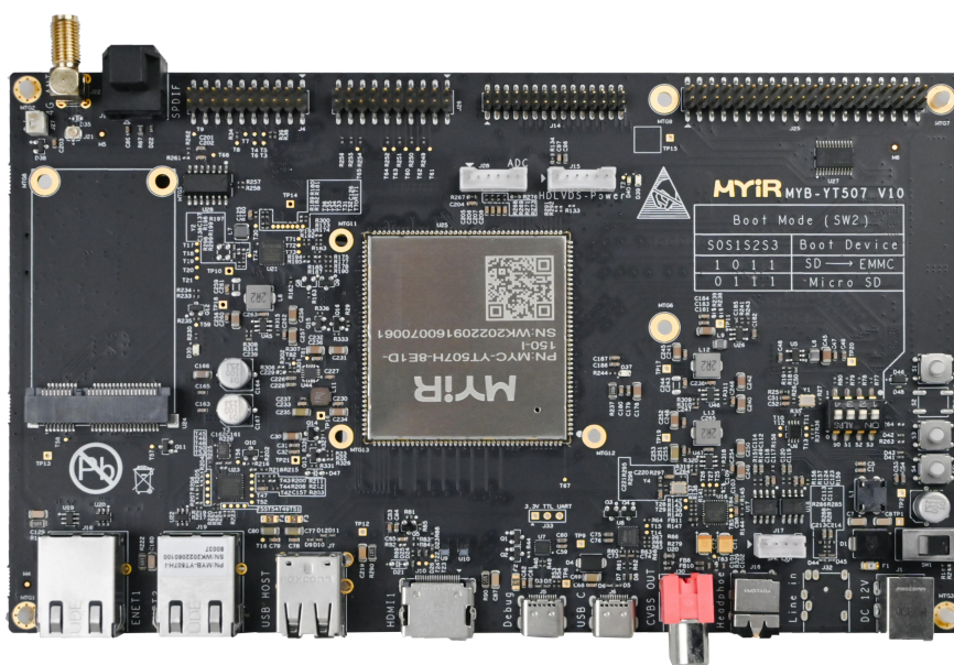
图 1-1 MYD-YT507H 开发板
