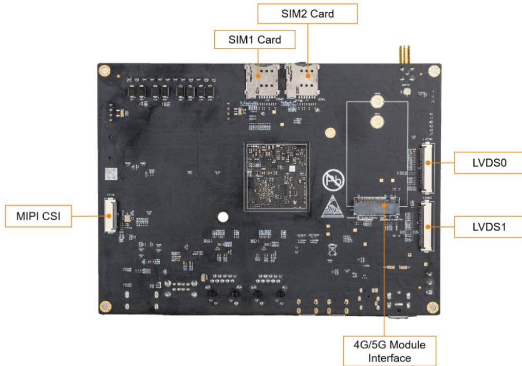
图 4-2 MYD-YM62X 开发板接口背面图
