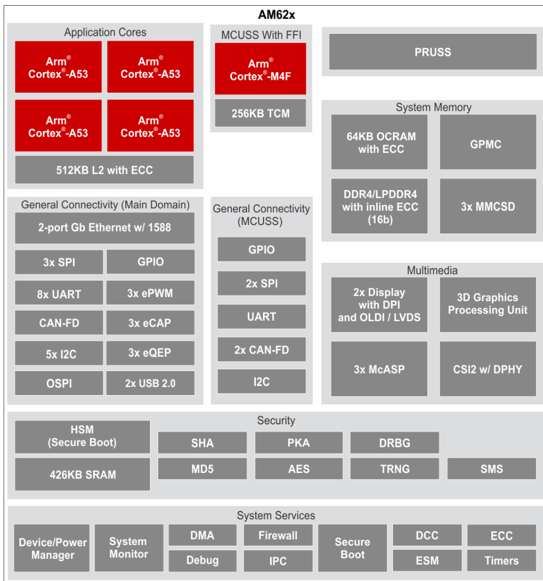
图 2-1 AM62x 处理器框图
