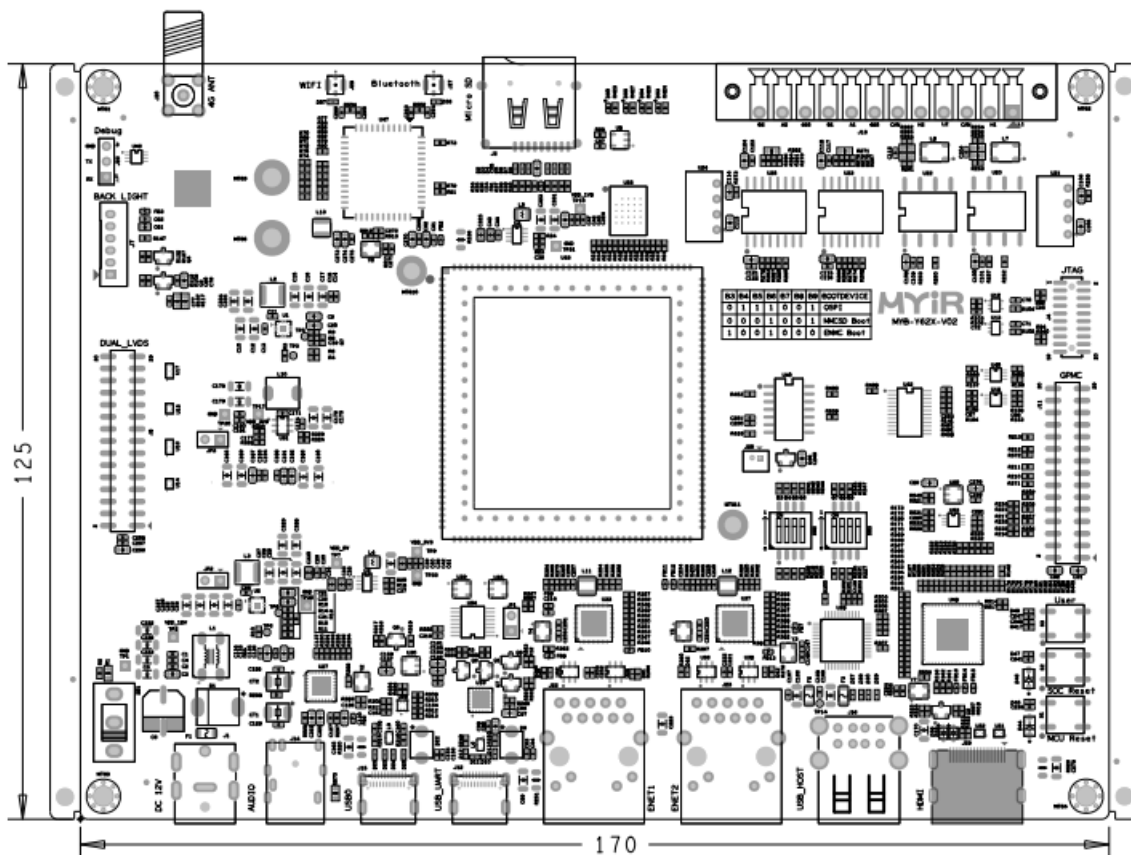
图 4-4 MYB-YM62X 机械尺寸图 (单位: mm)
