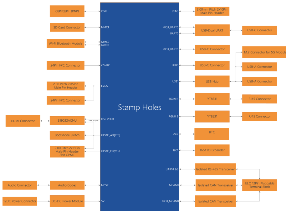
图 4-3 MYD-YM62X 开发板系统框架图
