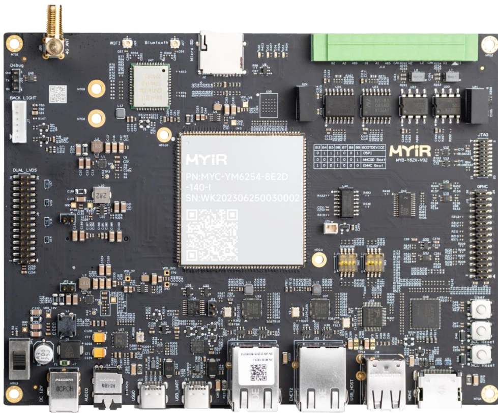
图 1-1 MYD-YM62X 开发板
