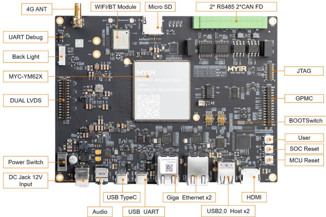
图 4-1 MYD-YM62X 开发板接口正面图
