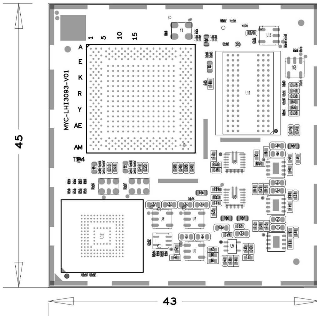
图 3-3 MYC-LHI3093 核心板机械结构图 (单位: mm)
