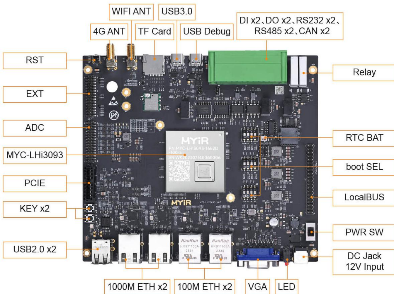
图 4-1 MYD-LHI3093 开发板接口正面图
