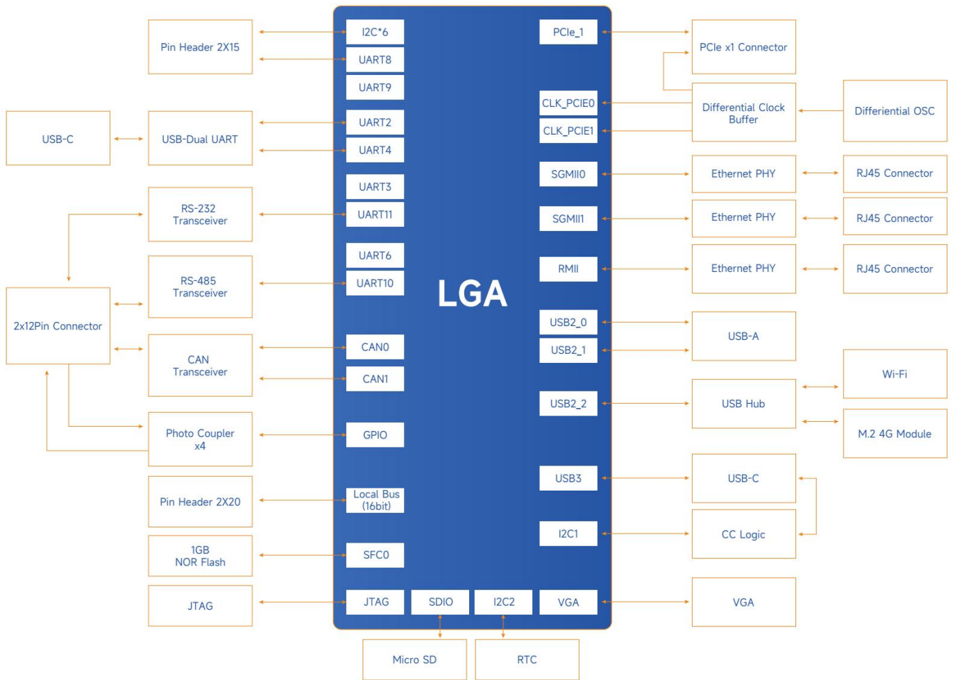
图 4-3 MYD-LHI3093 开发板系统框架图
