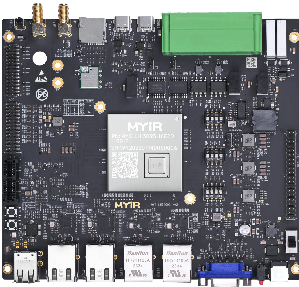
图 1-1 MYD-LHi3093 开发板
