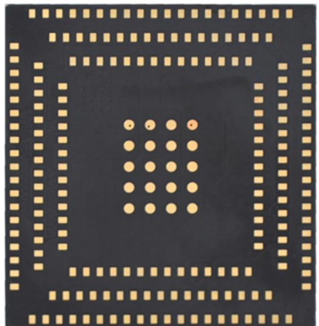
图 3-2 核心板 MYC-LMX9X 背面图
