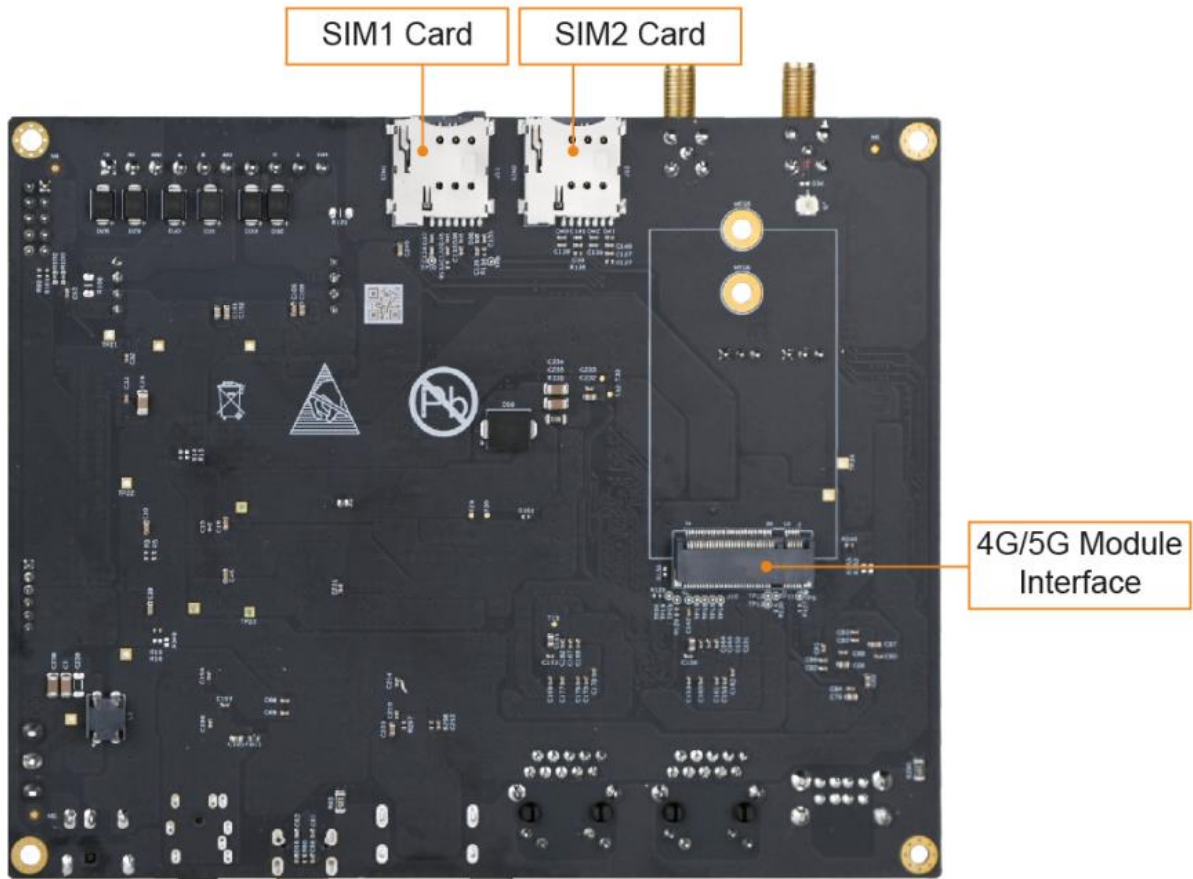
图 4-2 MYD-LMX9X 开发板接口背面接口图
