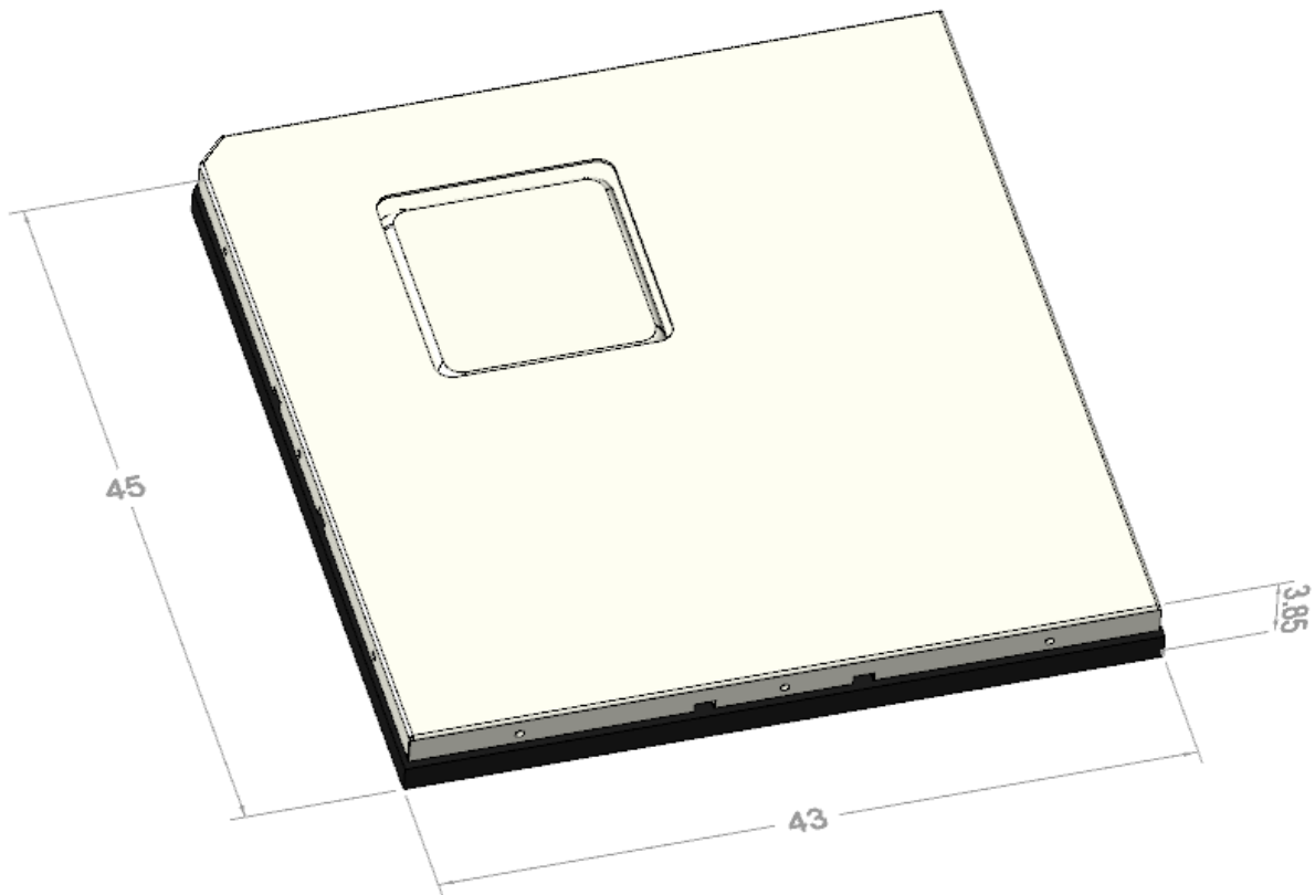
图 3-4 MYC-LT527 核心板机械结构图（单位：mm）
