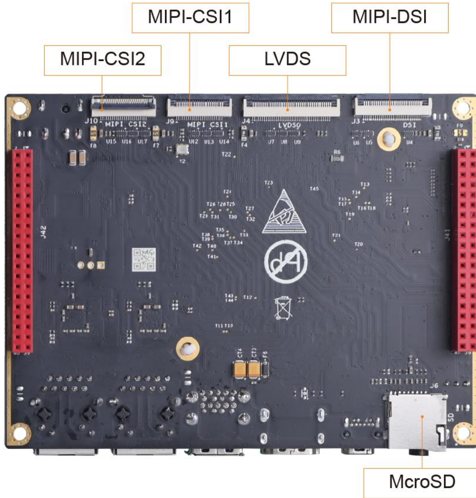
图 4-2 MYD-LT527 开发板接口背面图
