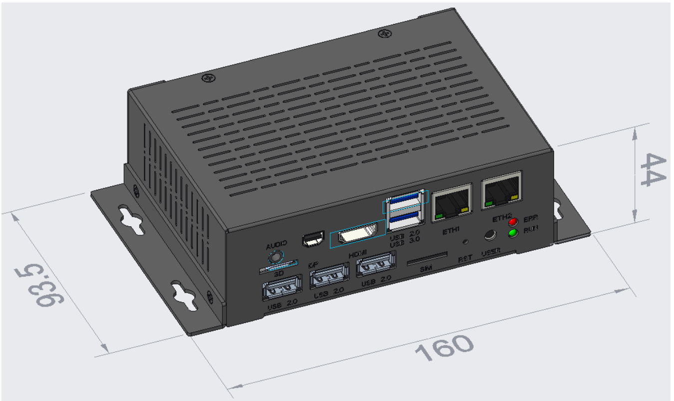
图 6-3 微型工控机机械尺寸图 (单位: mm)
