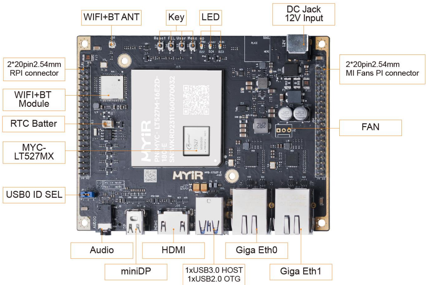
图 4-1 MYD-LT527 开发板接口正面图
