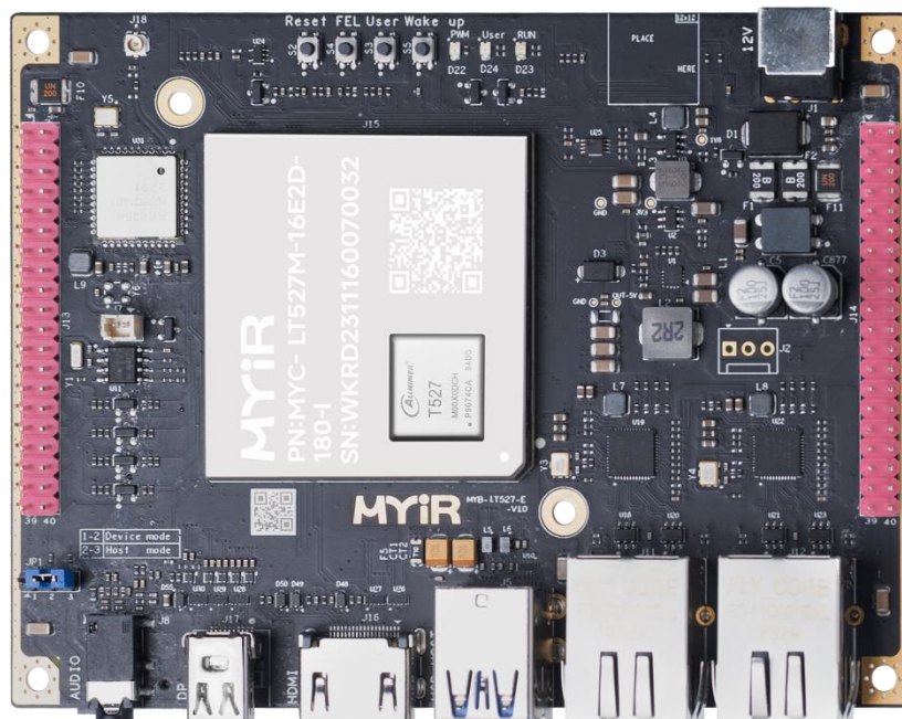
图 1-1 MYD-LT527 开发板
