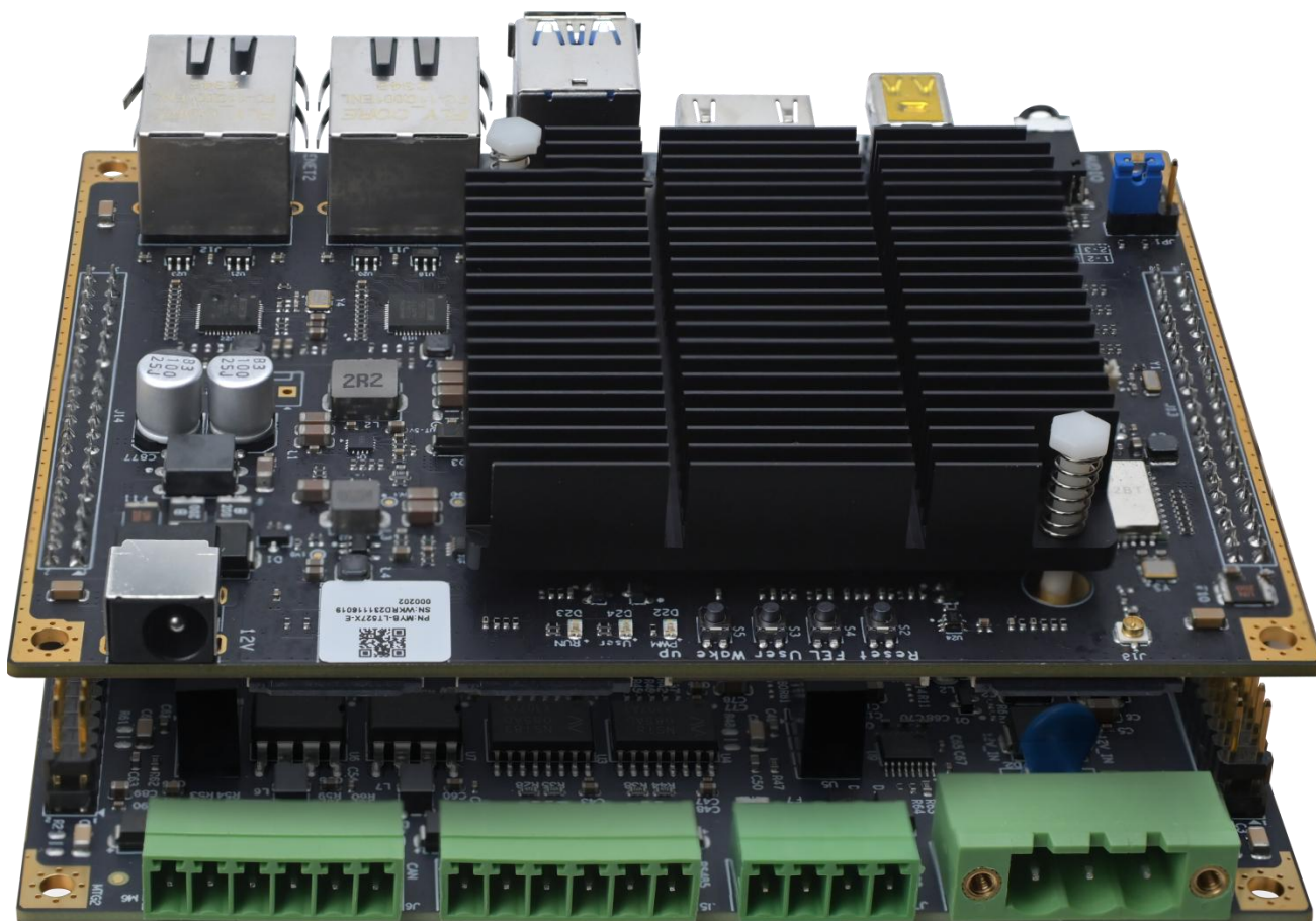
图 5-1 MYD-LT527-I-GK 工业开发板外观图
