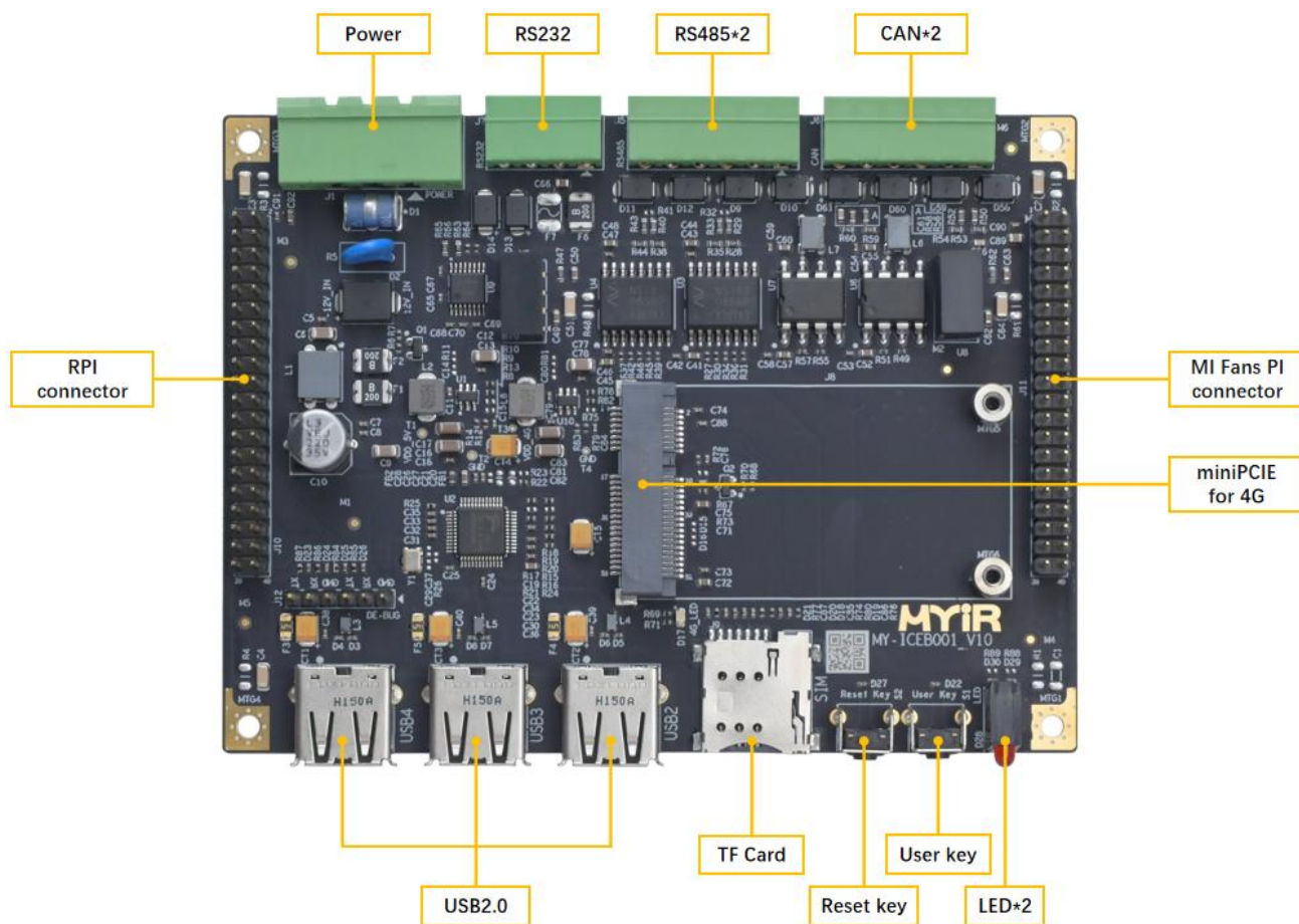
图 5-2 MYD-ICMB001 微型工控机扩展底板外观图
