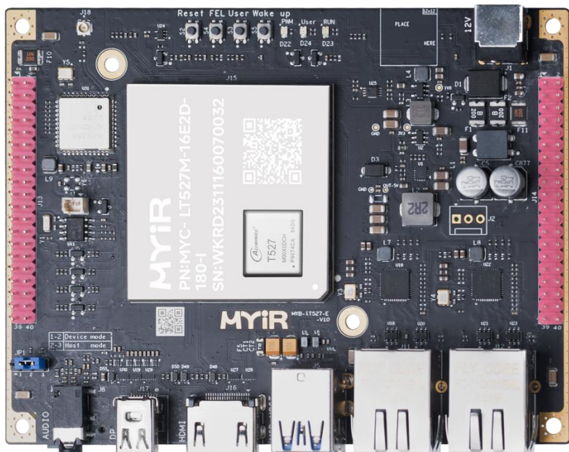
图 1-1 MYD-LT527 开发板
