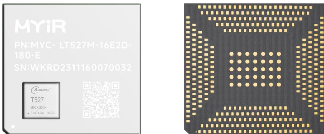
图 3-1 核心板 MYC-LT527 正反面图
