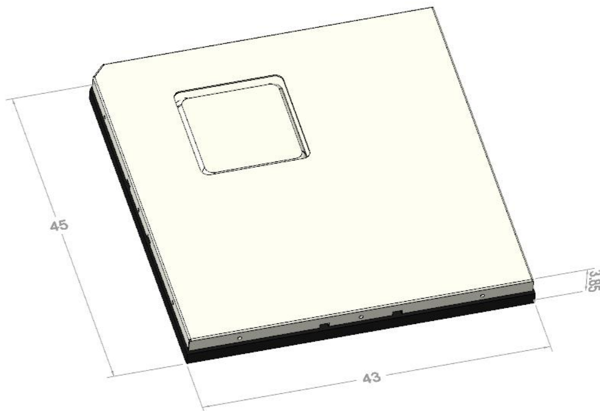
图 3-4 MYC-LT527 核心板机械结构图（单位：mm）
