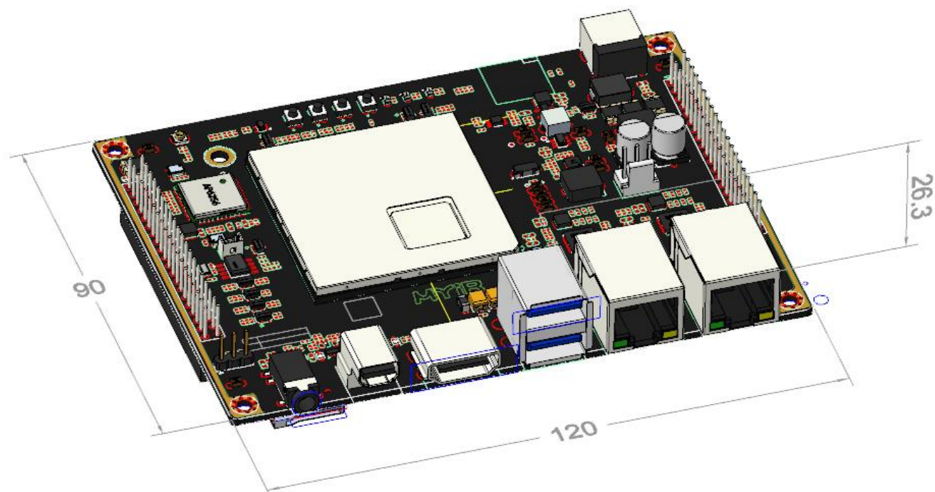
图 4-2 MYD-LT527 机械尺寸图 (单位: mm)
