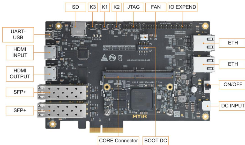
图 4-1 MYD-J7A100T 开发板接口正面图
