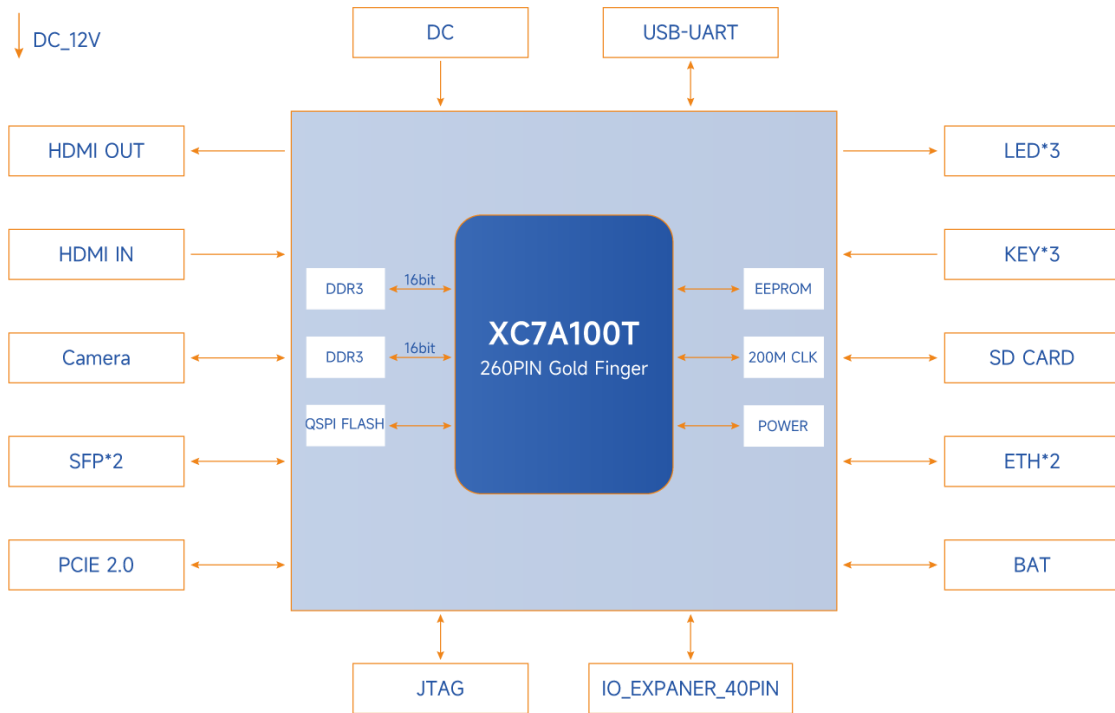
图 4-3 MYD-J7A100T 开发板系统框架图
