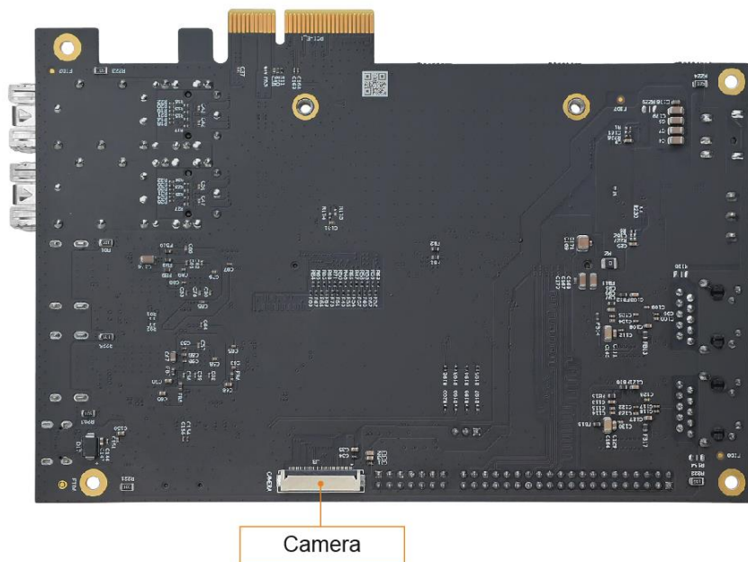
图 4-2 MYD-J7A100T 开发板接口背面接口图
