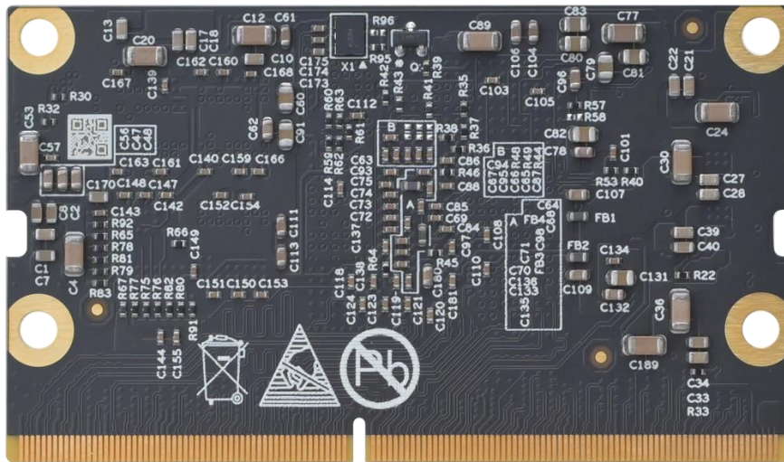
图 3-2 核心板 MYC-J7A100T 背面图
