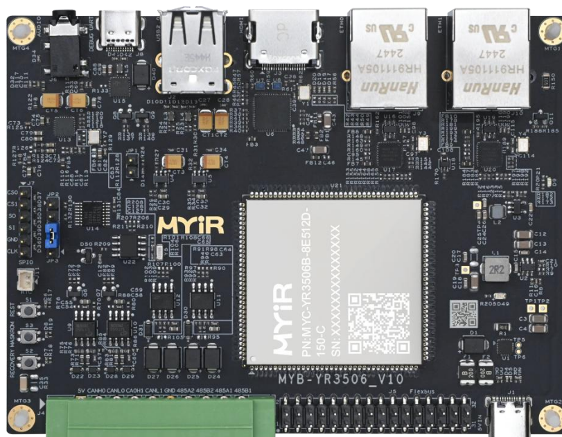
图 1-1 MYD-YR3506 开发板
