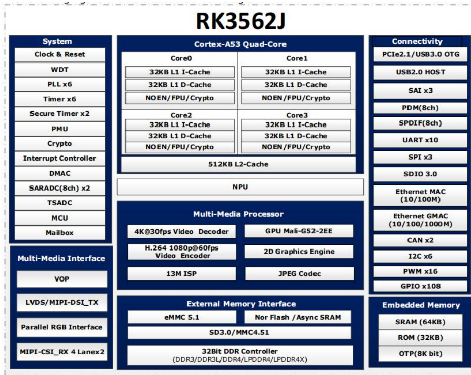
图 3-2 RK3562J 处理器框图
