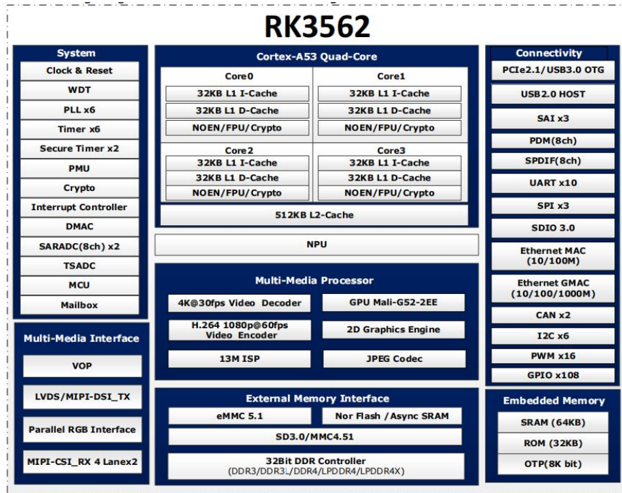
图 3-1 RK3562 处理器框图
